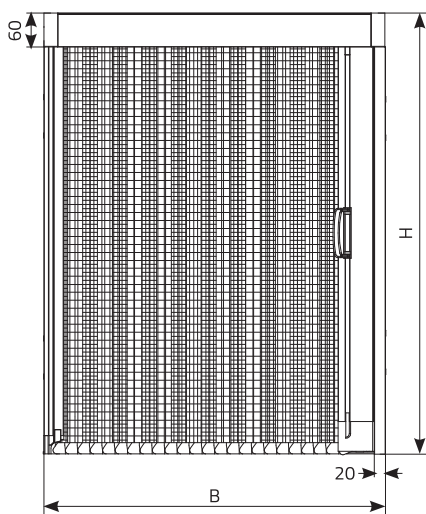
montaż: wnęka okienna
