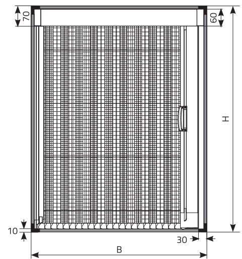
montaż: okno / fasada
