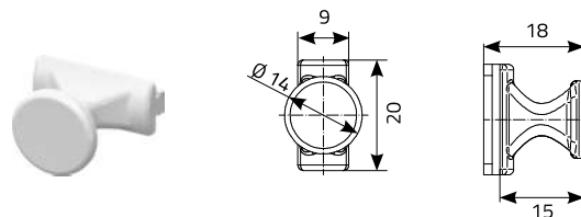
listwa hakowa dolna z odsadzeniem
