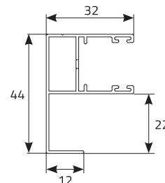
prowadnica z odsadzeniem (opcja za dopłatą)
