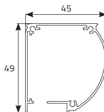
Przekrój skrzynki
