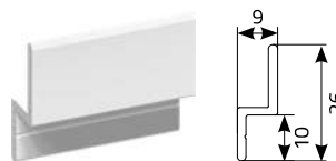
profil prowadnicy typ „Z”
