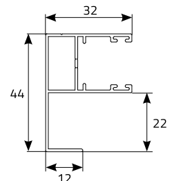
prowadnica z odsadzeniem (opcja za dopłatą)
